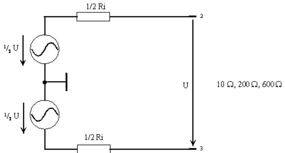
Bild 5-6: Channel = 1 oder 2
