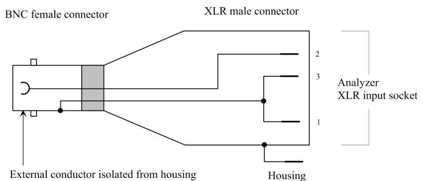
Bild 5-16: XLR/BNC-Adapter R&S UP-Z1M
