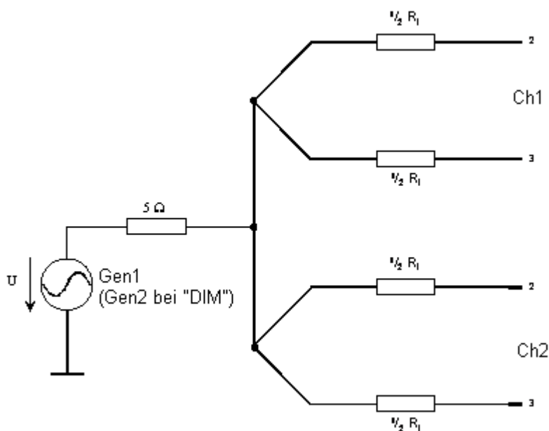
Bild 5-12: Channel 2 = 1
