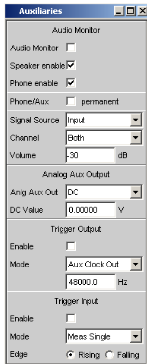
Bild 5-38: Bedienpanel Auxiliaries
