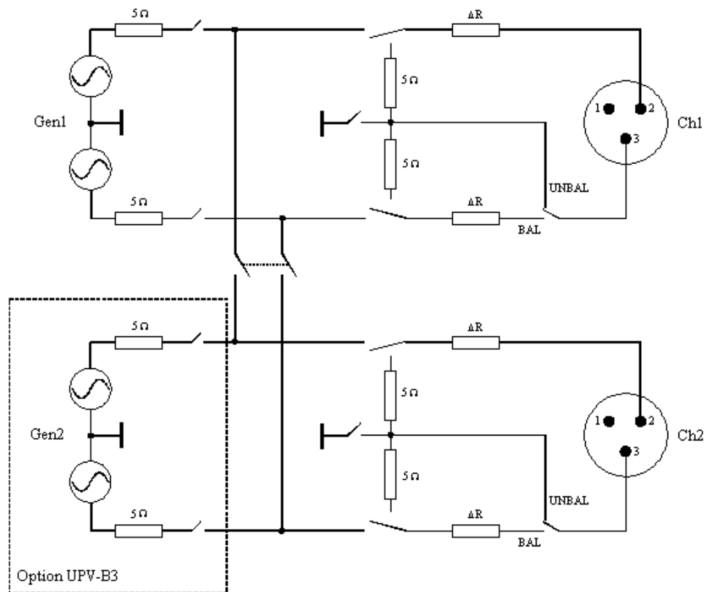
Bild 5-8: Beschaltung der Ausgänge bei Stereo Sine
