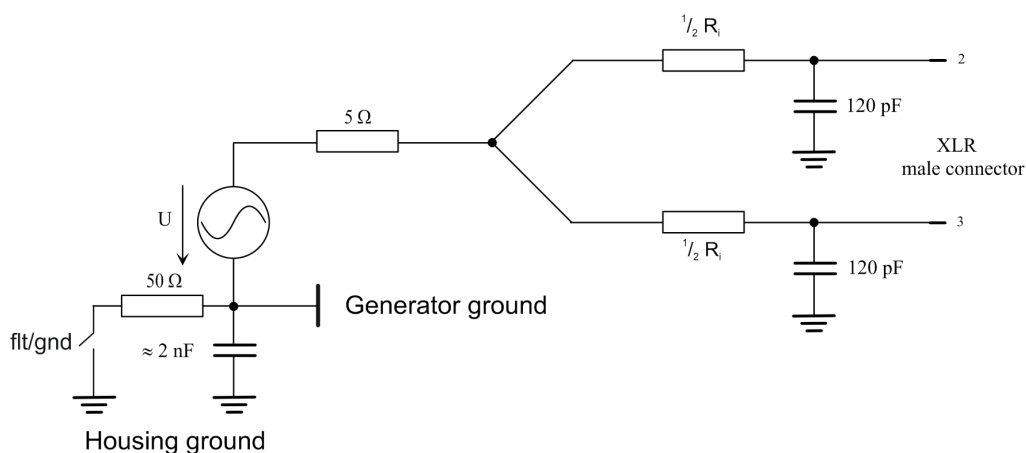
Bild 5-10: Ausgang mit Gleichtaktsignal
