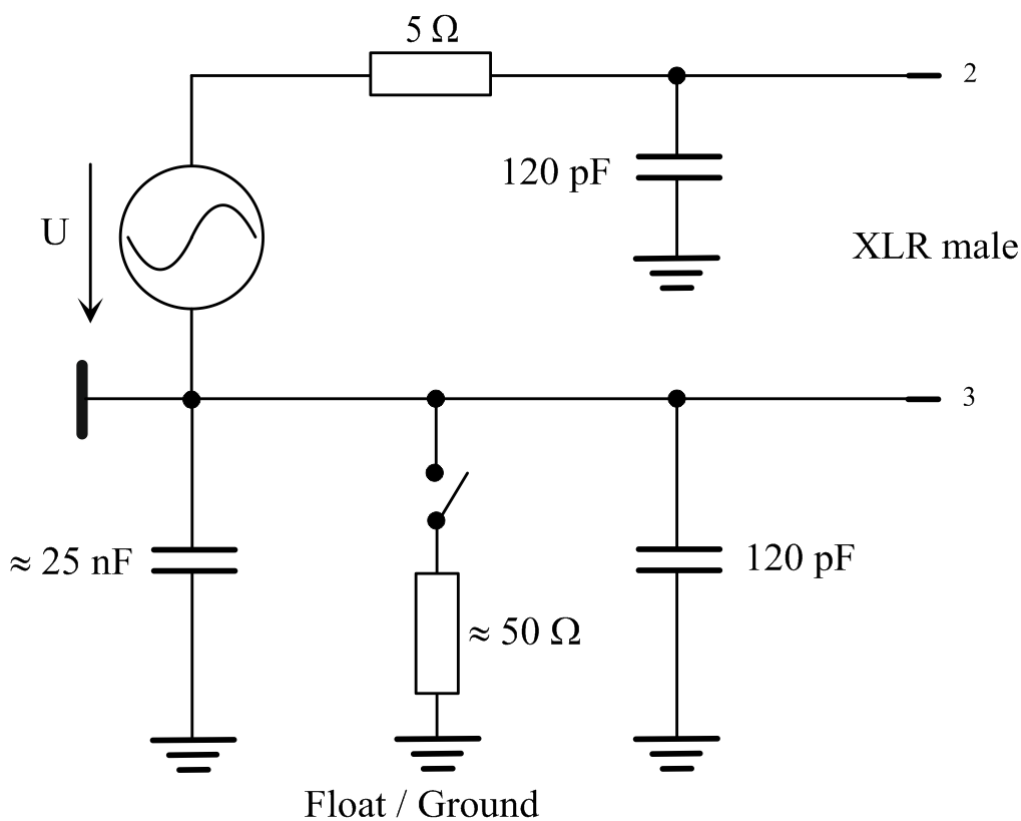
Bild 5-2: Unsymmetrischer Ausgang
