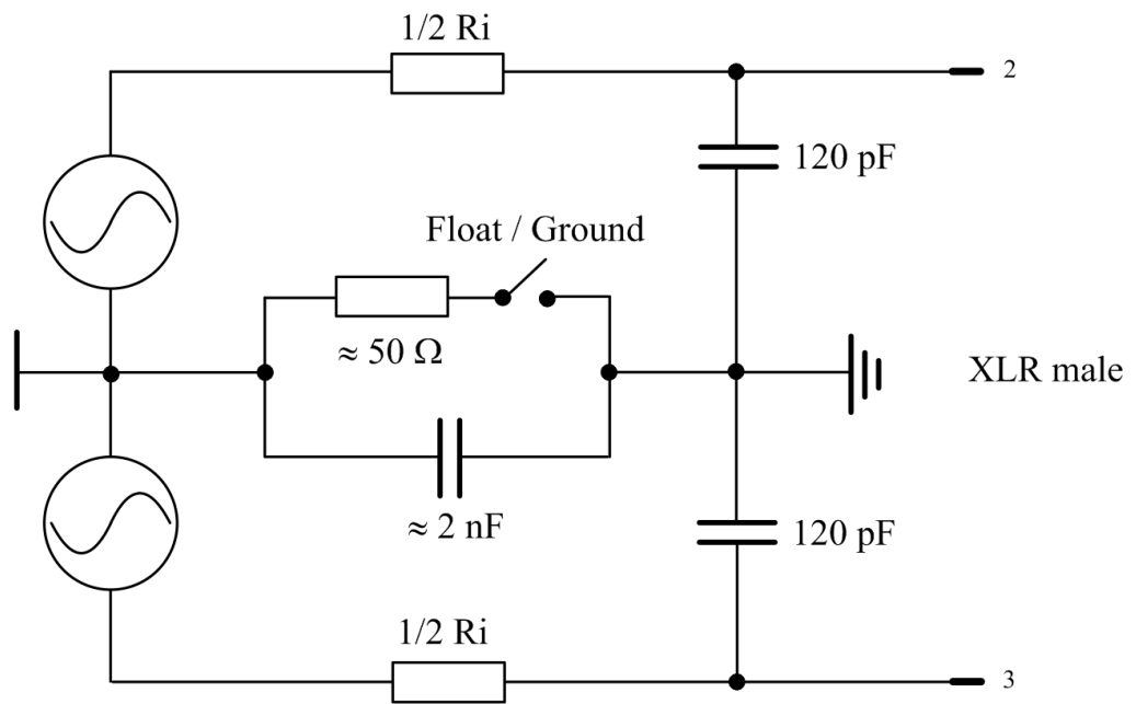
Bild 5-5: Symmetrischer Ausgang
