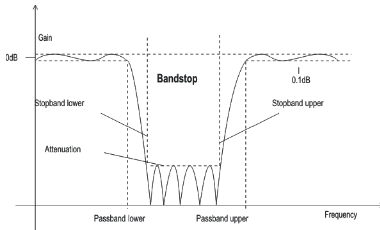
Bild 5-36: Band Stop Frequenzgang mit Kennzeichnung der Filterparameter
