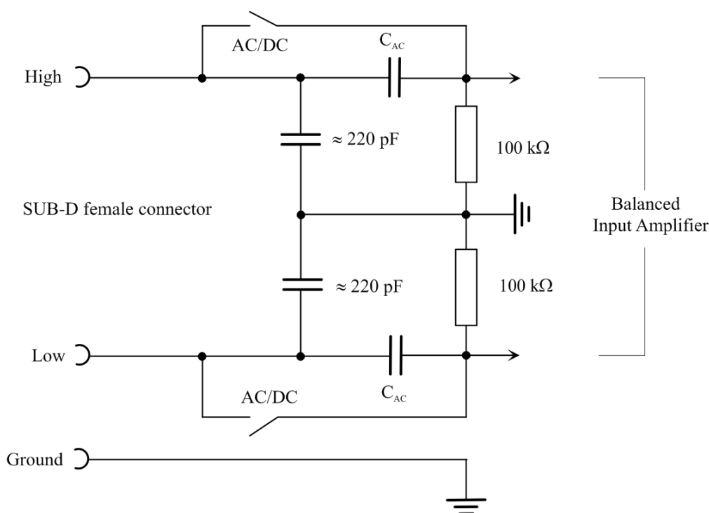
Bild 5-18: Symmetrischer Analyzer-Eingang
