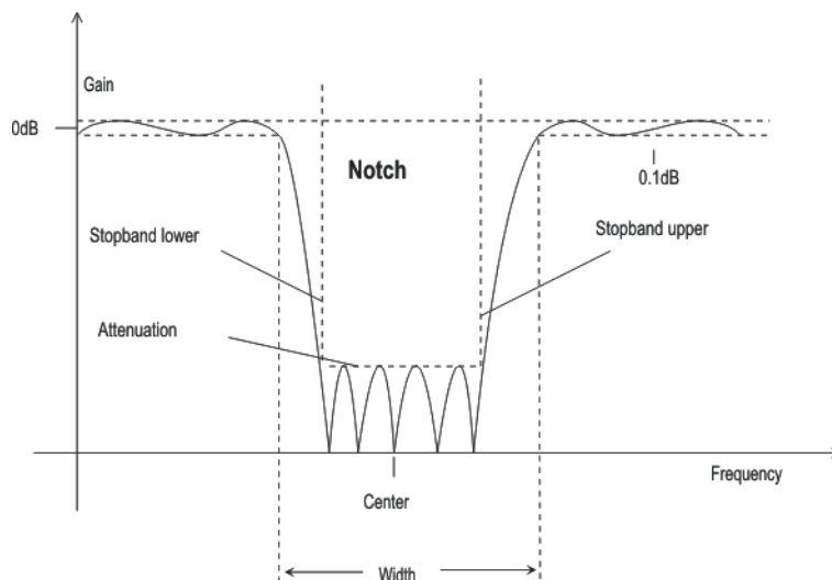
Bild 5-37: Notch-Filter Frequenzgang mit Kennzeichnung der Filterparameter
