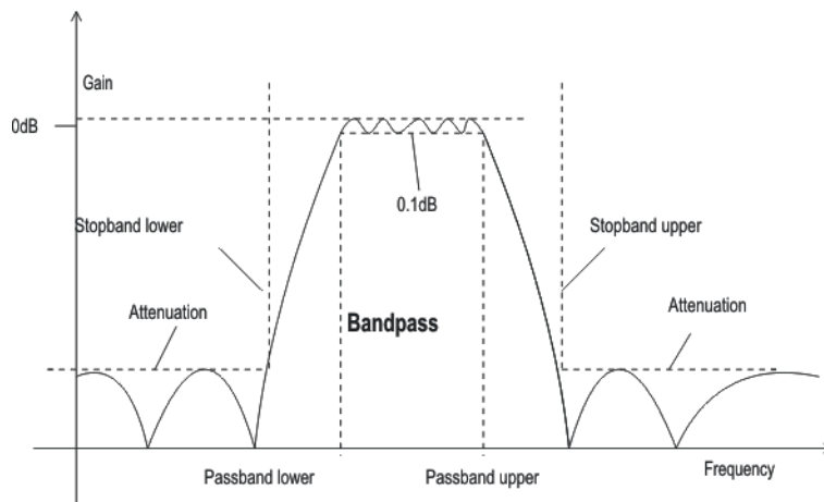
Bild 5-35: Band Pass Frequenzgang mit Kennzeichnung der Filterparameter
