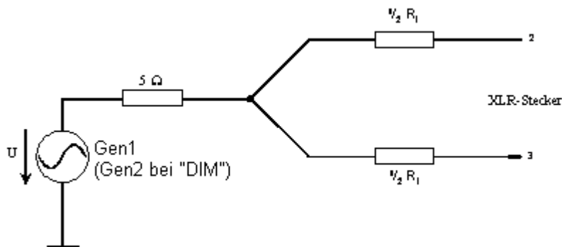
Bild 5-11: Channel 1 oder 2
