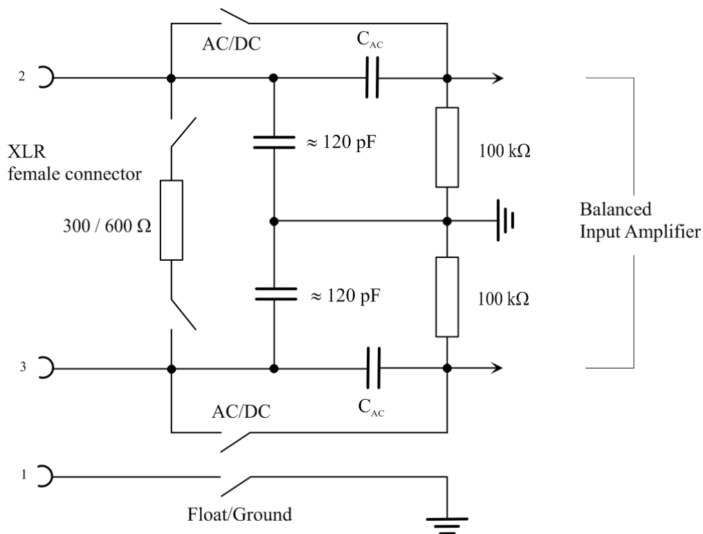
Bild 5-14: Symmetrischer Analyzer-Eingang
