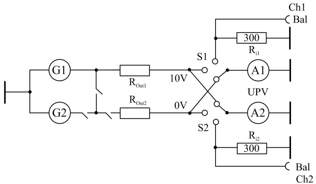
Bild 5-15: Verschaltungsmöglichkeiten der Analyzer-Eingänge
