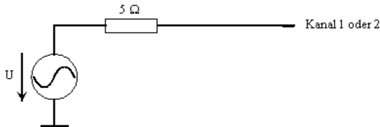
Bild 5-3: Channel = 1 oder 2
