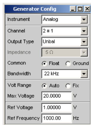
Bild 5-1: Konfigurationspanel Analog-Generator
